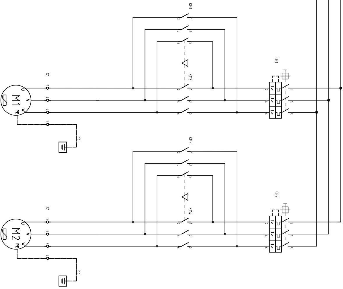
Электродвигатель задвижки 1
